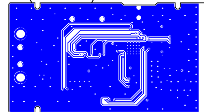
L4 (Scale 1:1)
