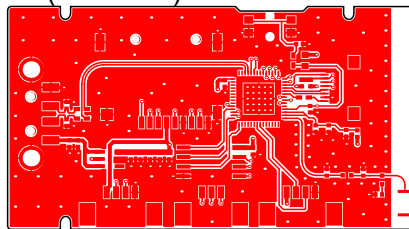
L1 (Scale 1:1)
